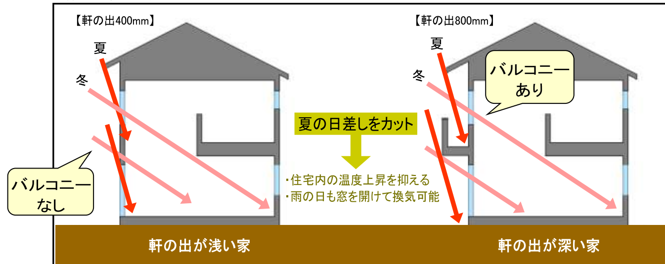
軒の出と光の入り方
